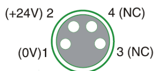
Bild2: M8-Stecker
